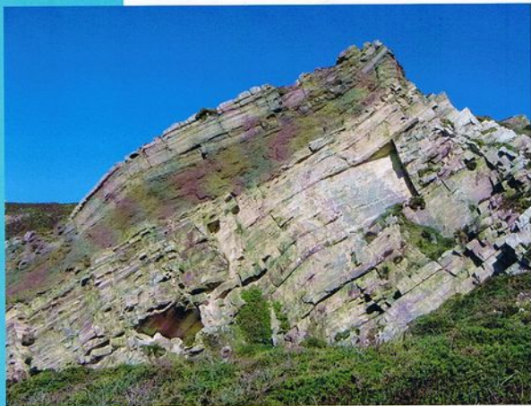
Coupe des formations détritiques du Paléozoïque Inférieur du Cap d'Erquy, Côtes d'Armor (photo C. Leprévost). Cf. article de Guy Lemasle, p. 43
